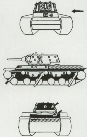
44-Tonner s.Pz.Kpfw. KW I verstärkt
