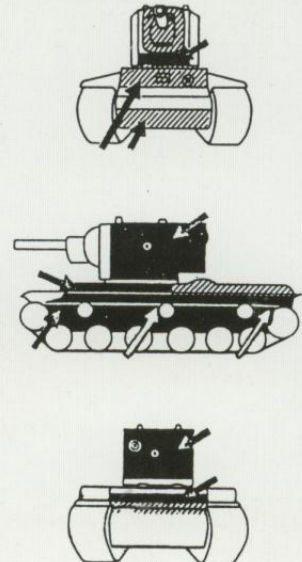
52-Tonner s.Pz.Kpfw. KW II
